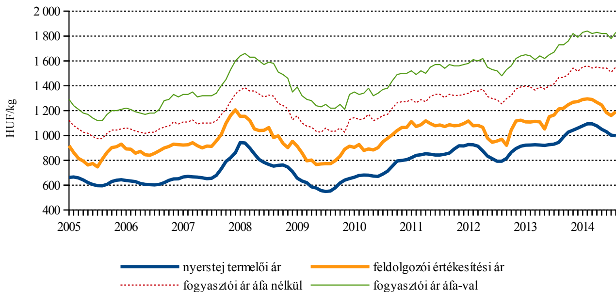
23. ábra: A Trappista sajt fázisárainak alakulása Magyarországon
